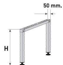
Montants inox avec vérins réglables
